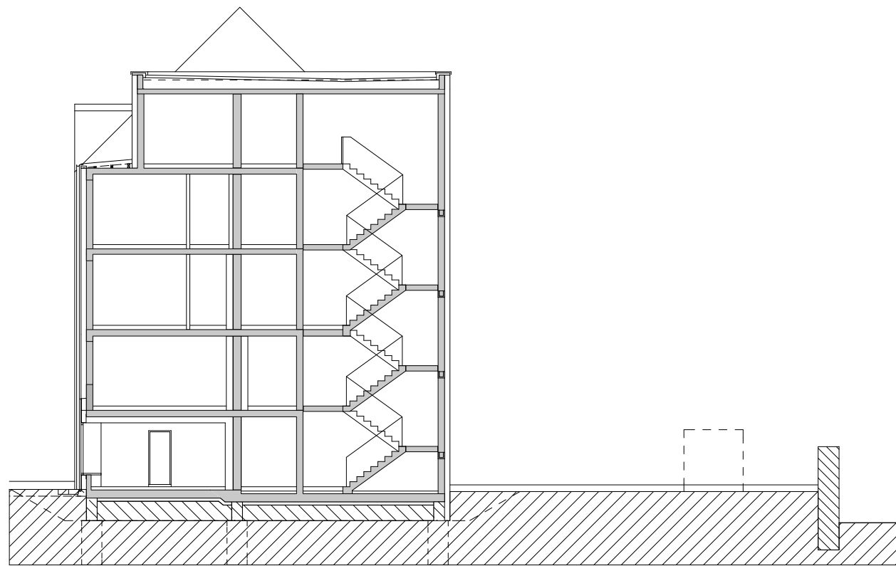
Querschnitt C-C
