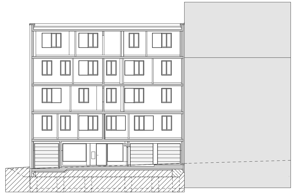
Querschnitt A-A
