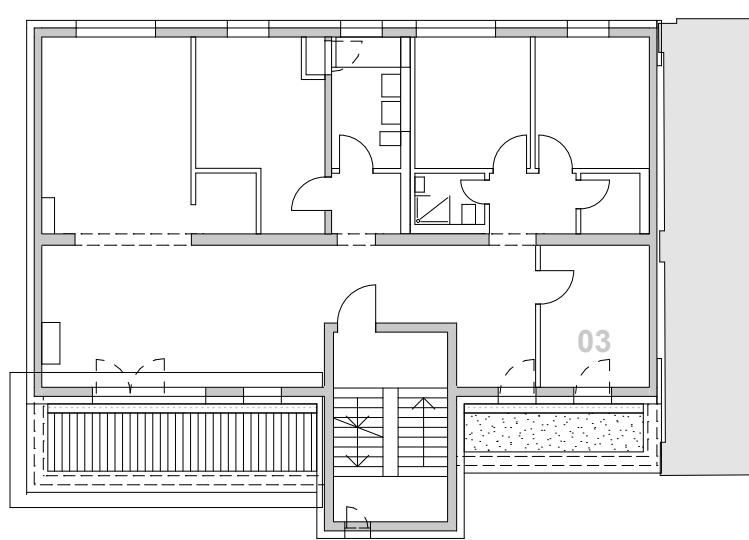
2.Obergeschoss
