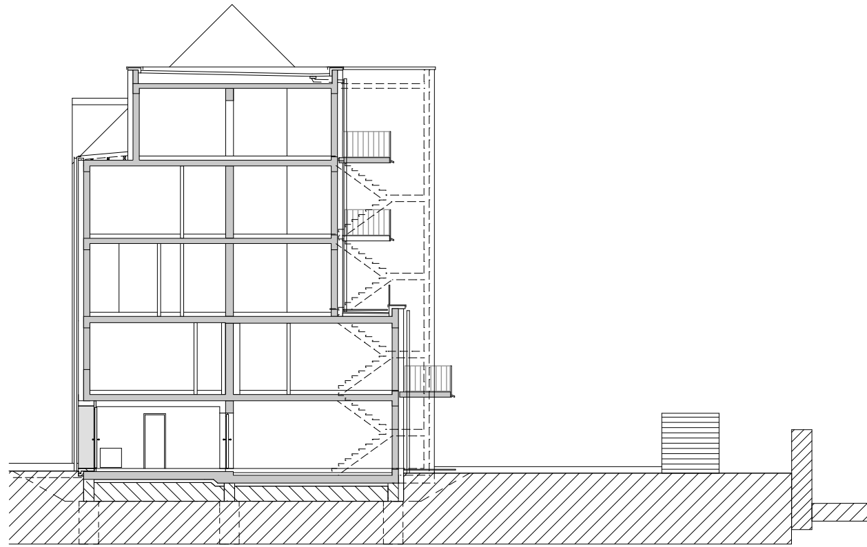
Querschnitt A-A
