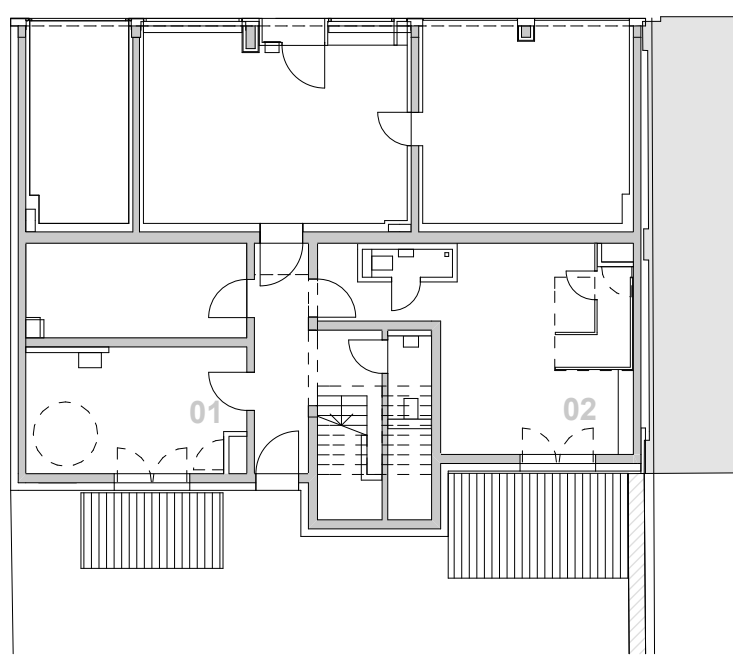
Erdgeschoss
