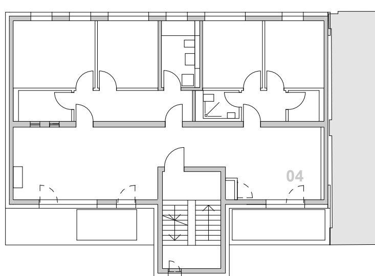
3.Obergeschoss
